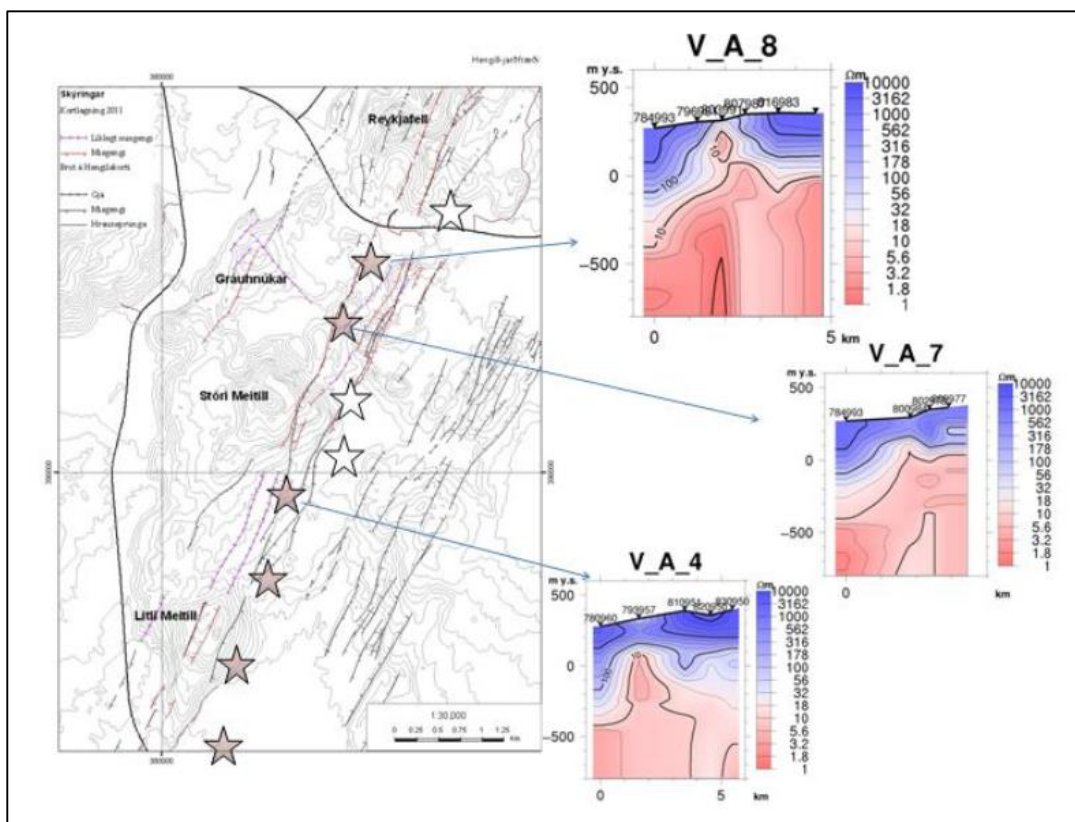
Mynd 5. Jarðeðlisfræðileg gögn yfirfærð á sprungu/misgengiskort (Björn S. Harðarson og Sigurður G. Kristinsson, 2012)
