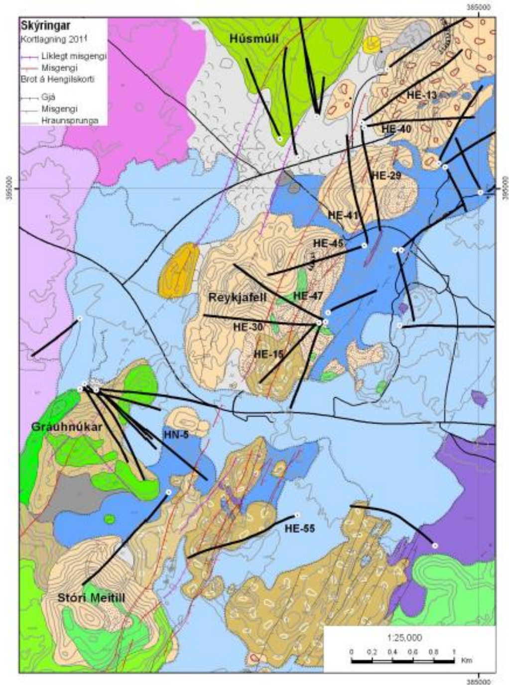
Mynd 4. Jarðfræðikort af Gráuhnúkasvæðinu sem nær suður fyrir Stóra-Meitill (Björn S. Harðarson og Sigurður G. Kristinsson, 2012)
