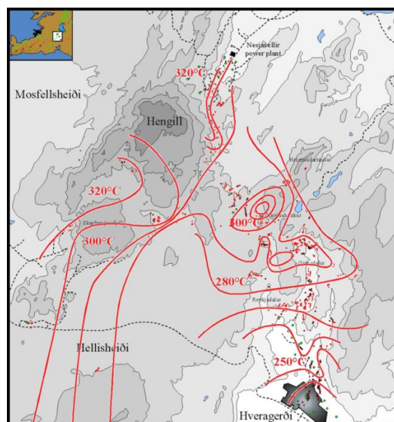
Mynd 4. Dreifing gashita á Hengilssvæði (Gretar Ívarsson, 1998)
