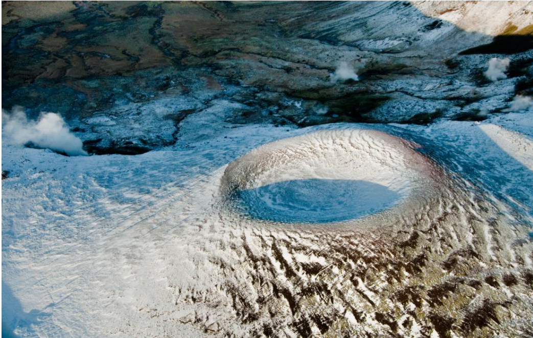
Mynd 3. Tjarnarhnúkur og jarðhiti í Lakaskörðum
