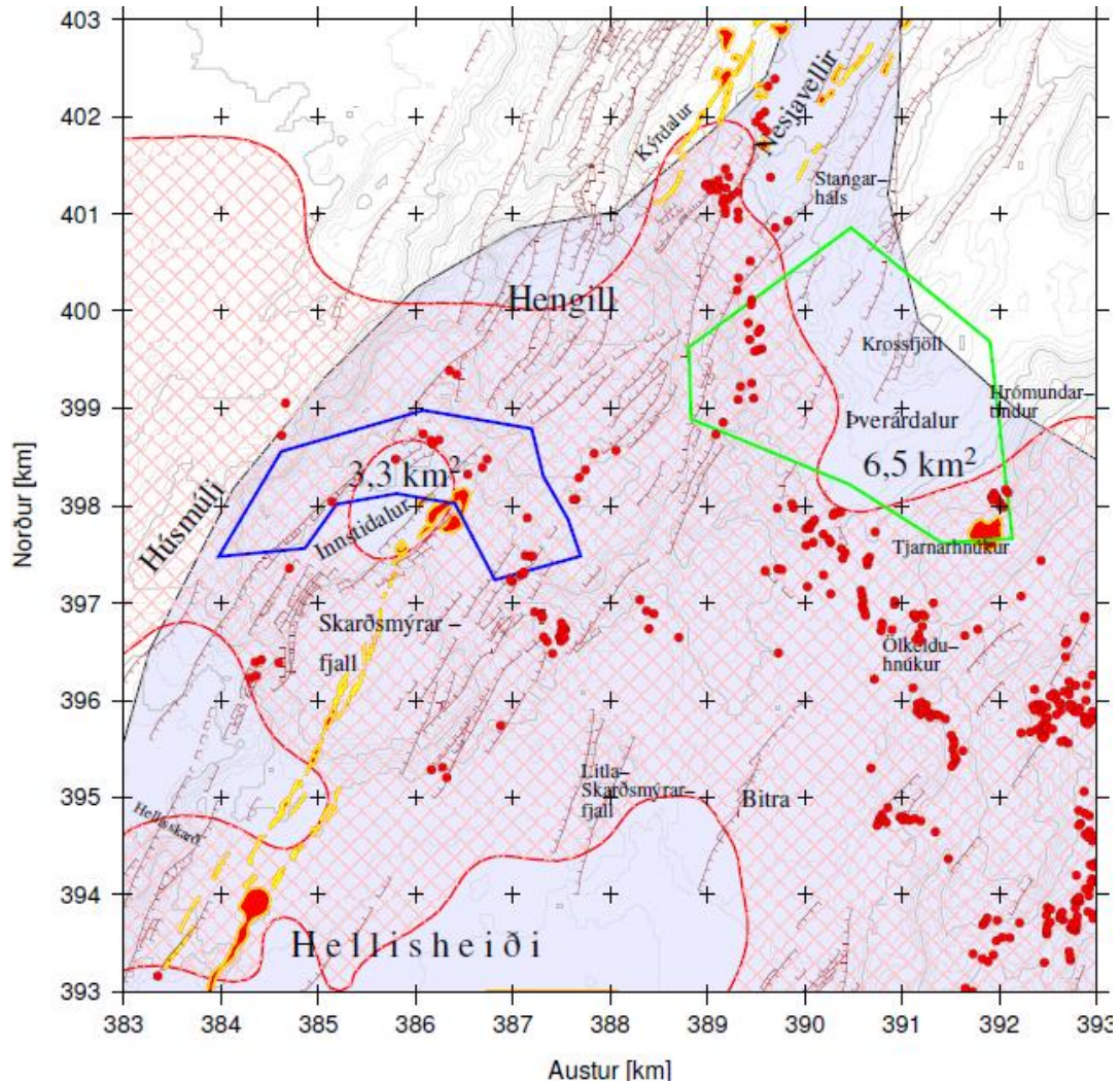
Mynd 6. Dreifing lágviðnáms og háviðnámskjarna á norður hluta Hengillssvæðisins (Gunnar Gunnarsson óbirt kort)
