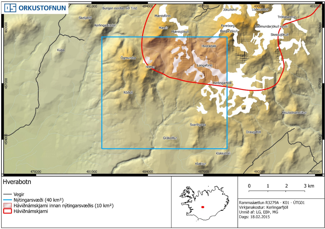
Mynd 4-3: Hverabotn, kort sem sýnir hugsanlegt nýtingarsvæði.
