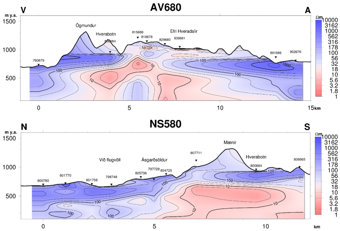
Mynd 4-3: Viðnámssnið af Hverabotni (Ragna Karlsdóttir o.fl., 2010).
