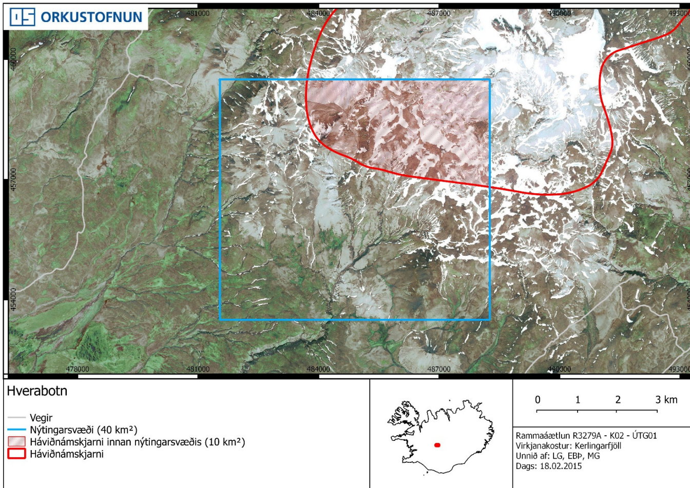
Mynd 4-4: Hverabotn, lofimynd sem sýnir hugsanlegt nýtingarsvæði.
