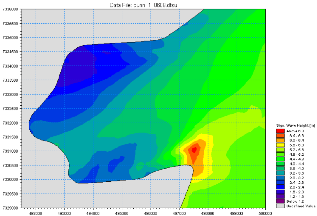
Mynd 33 Alda úr norðaustri með 100 ára endurkomutíma – H_s = 10,6m , T_p = 14,7s
