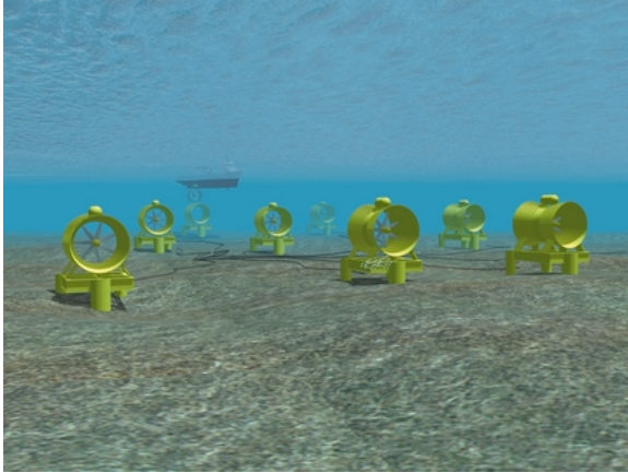
Mynd 24: Teikning af hugmynd Lunar Energy um sjávarvirkjun á hafsbotni.
