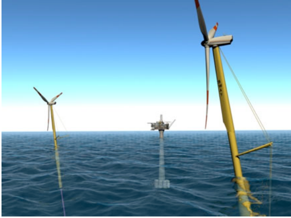
Mynd 10: Fljótandi framtíðarvindorkuver úti á sjó; hugmynd norska fyrirtækisins Sway í samstarfi við NorskHydro.
