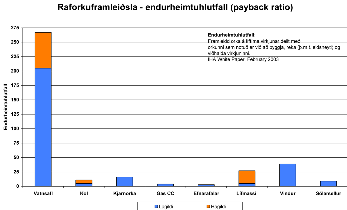
Mynd 23: Endurheimtuhlutfall mismunandi tegunda af raforkuframleiðslu.
